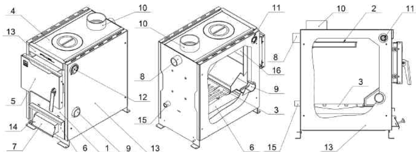
Рис. 1 Устройство котла
